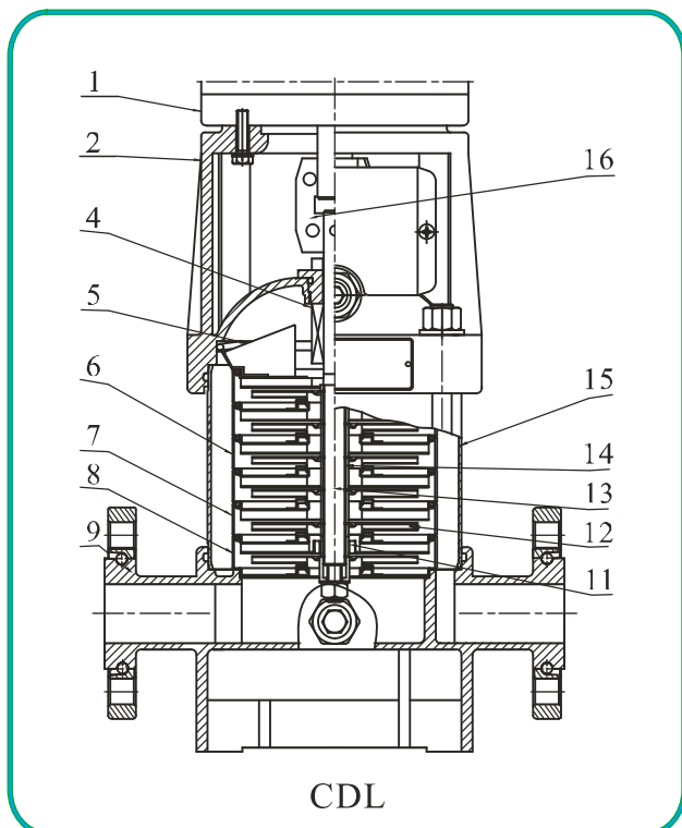
截面图 CDL,CDLF1,2,3,4
